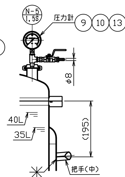
A部詳細図 S = 1 : 3
