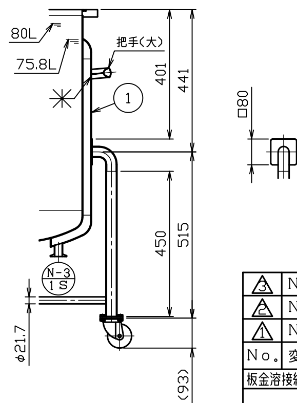
ドレン部詳細図 S = 1 : 5
