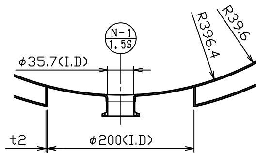
ドレン部詳細図 S = 1 : 5
