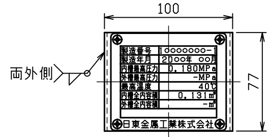
銘板詳細図 S = 1 : 3
