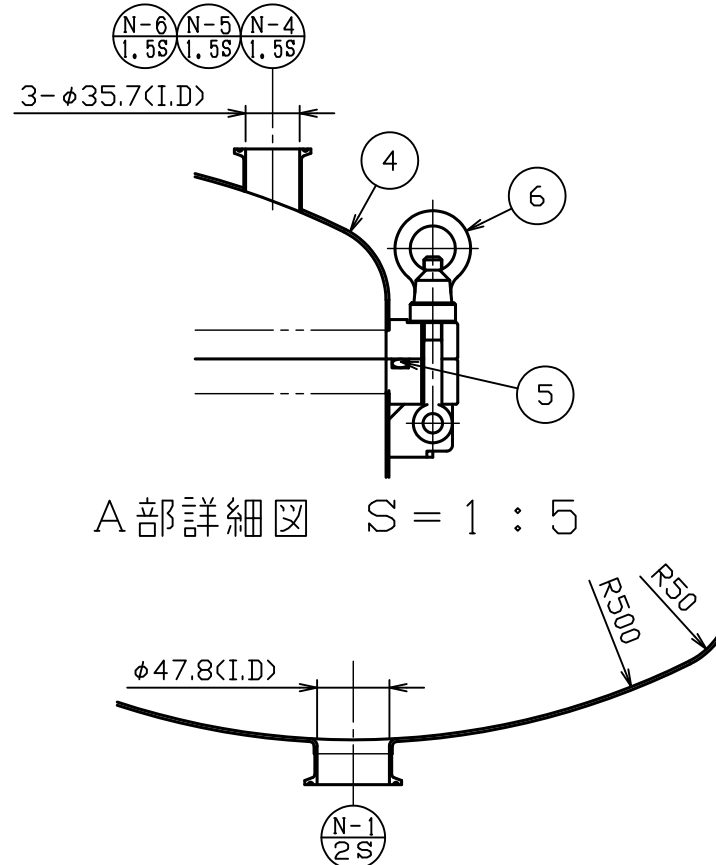
ドレン部詳細図 S = 1 : 5
