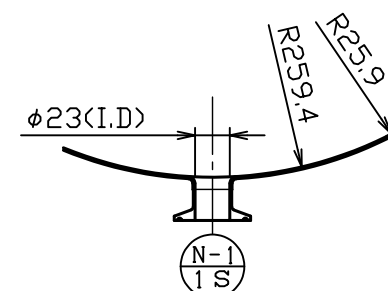
ドレン部詳細図 S = 1 : 5
