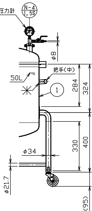
ドレン部詳細図 S = 1 : 5
