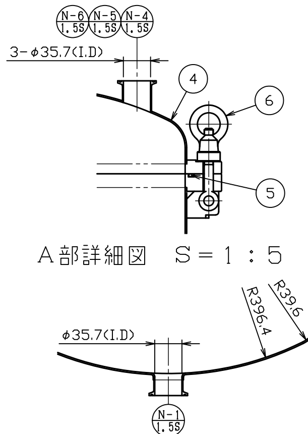
ドレン部詳細図 S = 1 : 5
