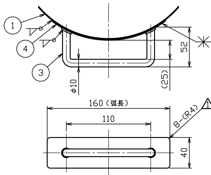
把手部詳細図 S = 1 : 3
