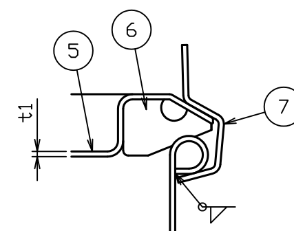
A部詳細図 S = 1 : 1
