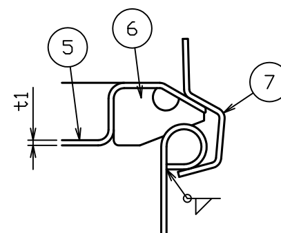
A部詳細図 S = 1 : 1
