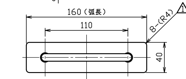
把手部詳細図 S = 1 : 3
