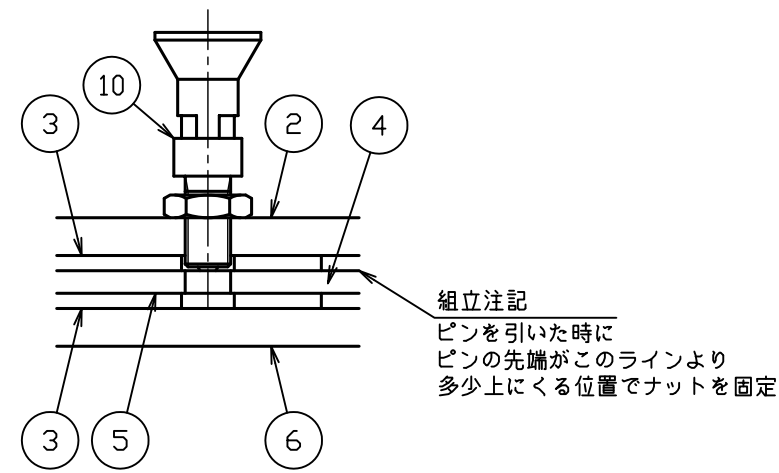
A 部詳細図 S = 1 : 1
