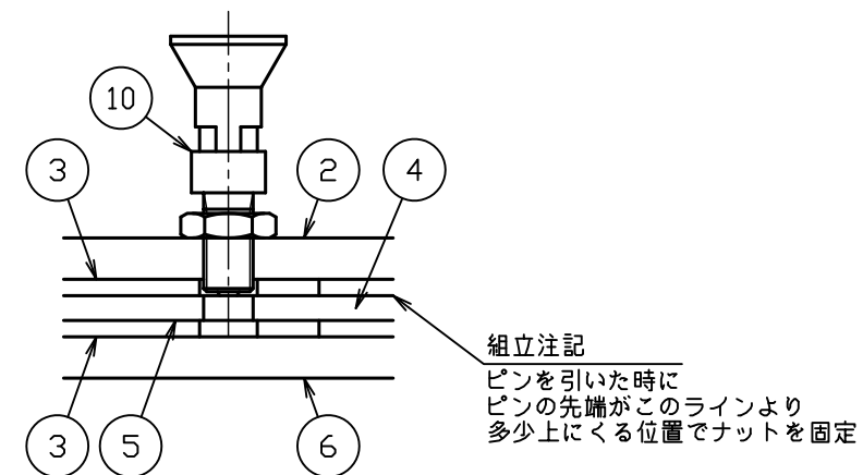
△ A部詳細図 S = 1 : 1
