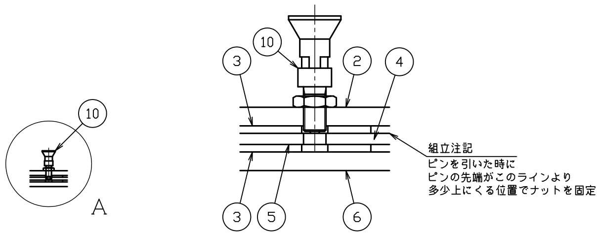
A部詳細図 S = 1 : 1
