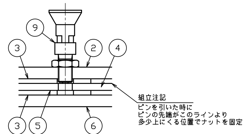
A部詳細図 S = 1 : 1
