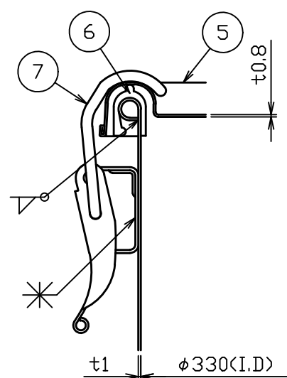
B部詳細図 S = 1 : 2
