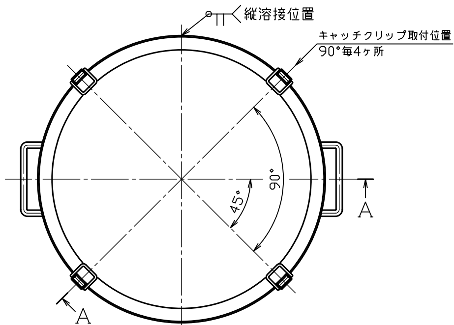
B部詳細図 S = 1 : 2
