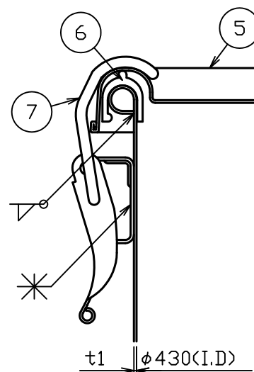
B部詳細図 S = 1 : 2
