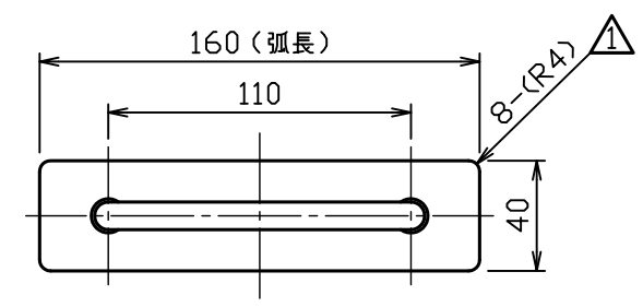
把手部詳細図 S = 1 : 3
