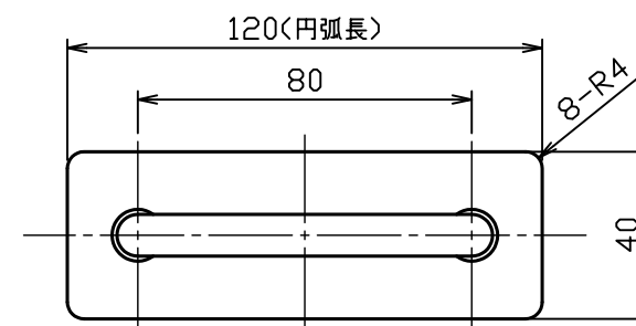
把手部詳細図 S = 1 : 2
