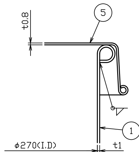
A部詳細図 S = 1 : 1
