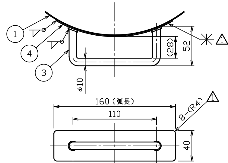
把手部詳細図 S = 1 : 3
