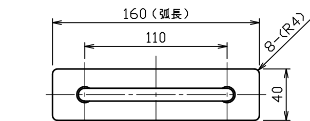
把手部詳細図 S = 1 : 3
