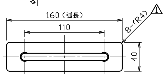
把手部詳細図 S = 1 : 3
