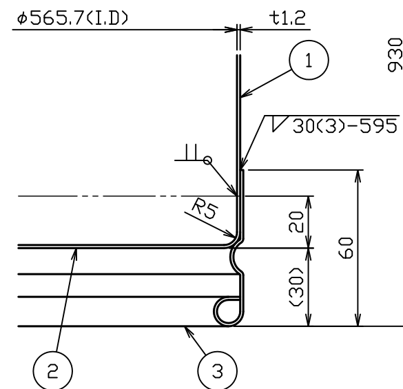
A部詳細図 S = 1 : 2
