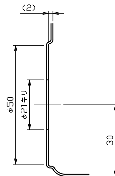
エンボス加工詳細図 S = 1 : 1
