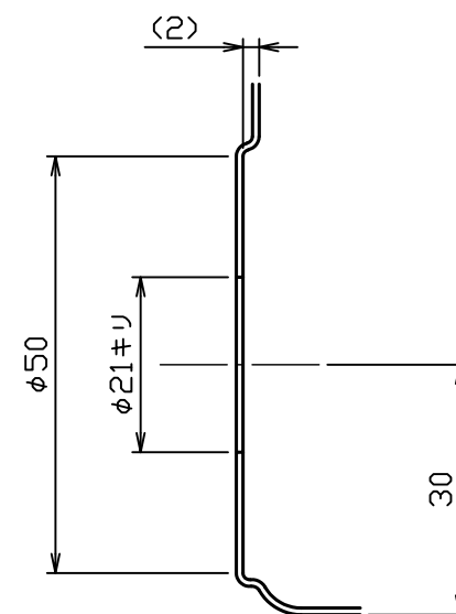
エンボス加工詳細図 S = 1 : 1
