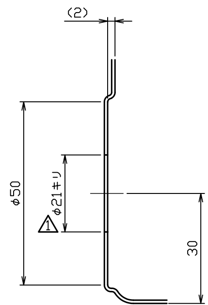
エンボス加工詳細図 S = 1 : 1
