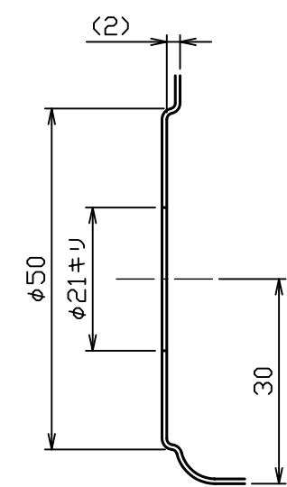
エンボス加工詳細図 S = 1 : 1
