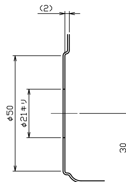
エンボス加工詳細図 S = 1 : 1
