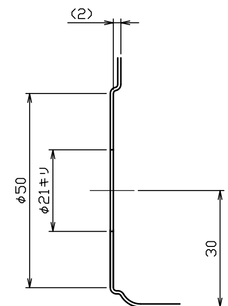
エンボス加工詳細図 S = 1 : 1
