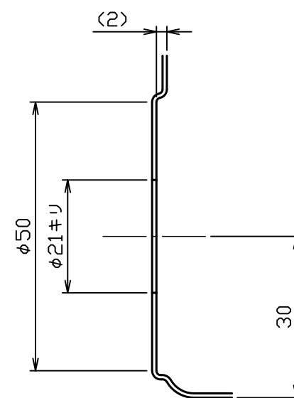
エンボス加工詳細図 S = 1 : 1
