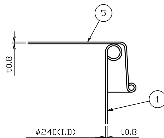
A部詳細図 S = 1 : 1
