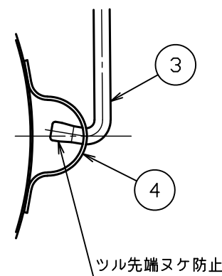
△△ B部詳細図 S = 1 : 2
