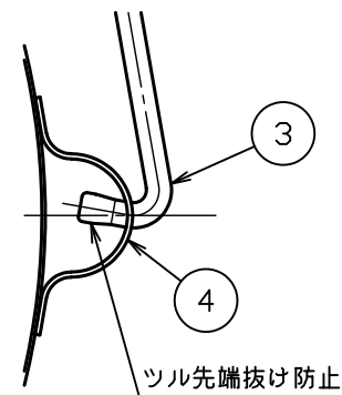
△△ A部詳細図 S = 1 : 2
