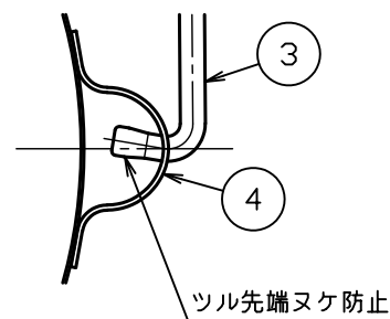
△△ A部詳細図 S = 1 : 2
