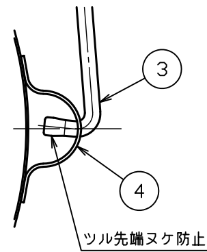
△ A 部詳細図 S = 1 : 2
