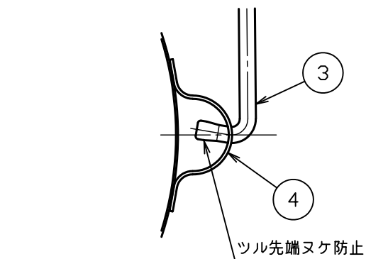
△A部詳細図 S = 1 : 2
