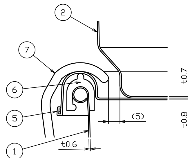
積み重ね詳細図 S = 1 : 1
