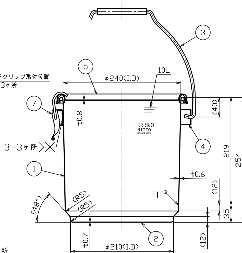
A-A断面図
