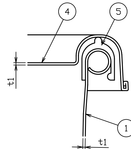
A部詳細図 S = 1 : 1
