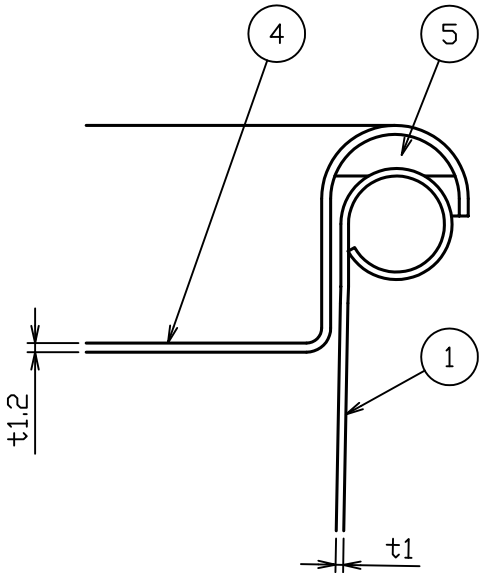
A部詳細図 S = 1 : 1
