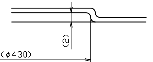
B部詳細図 S = 2 : 1
