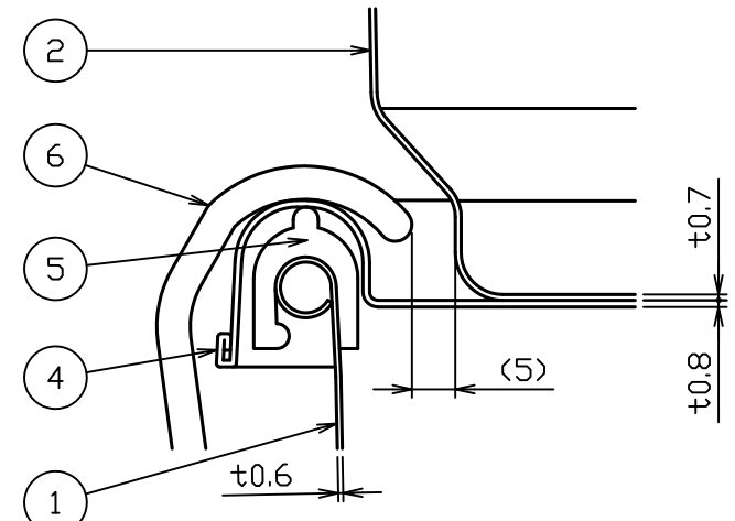
積み重ね詳細図 S = 1 : 1
