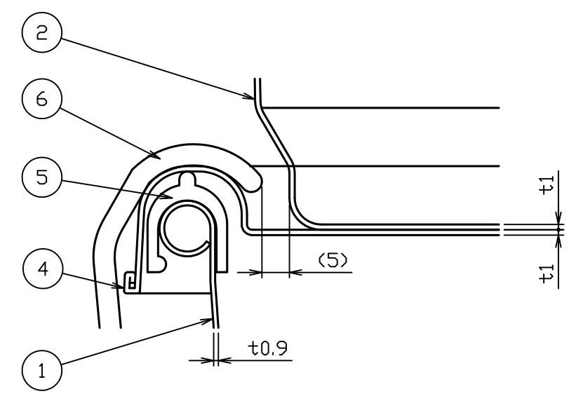
積み重ね詳細図 S = 1 : 1
