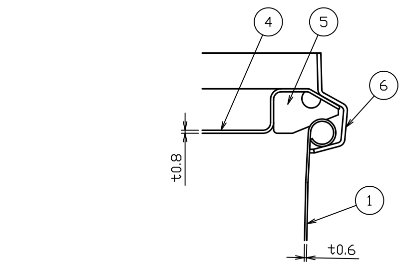
A部詳細図 S = 1 : 1
