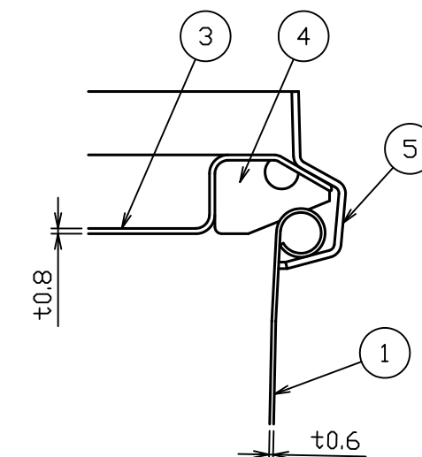
A部詳細図 S = 1 : 1
