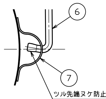
△ B部詳細図 S = 1 : 2
