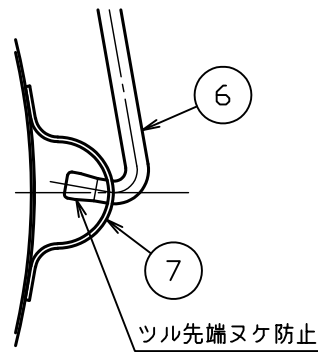
△ B部詳細図 S = 1 : 2
