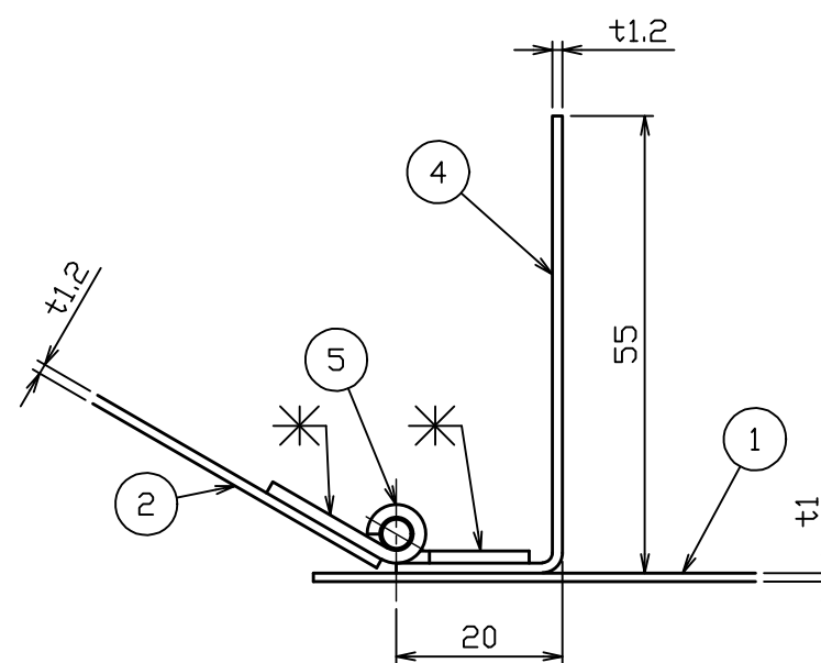
蝶番取付詳細図 S = 1 : 1
