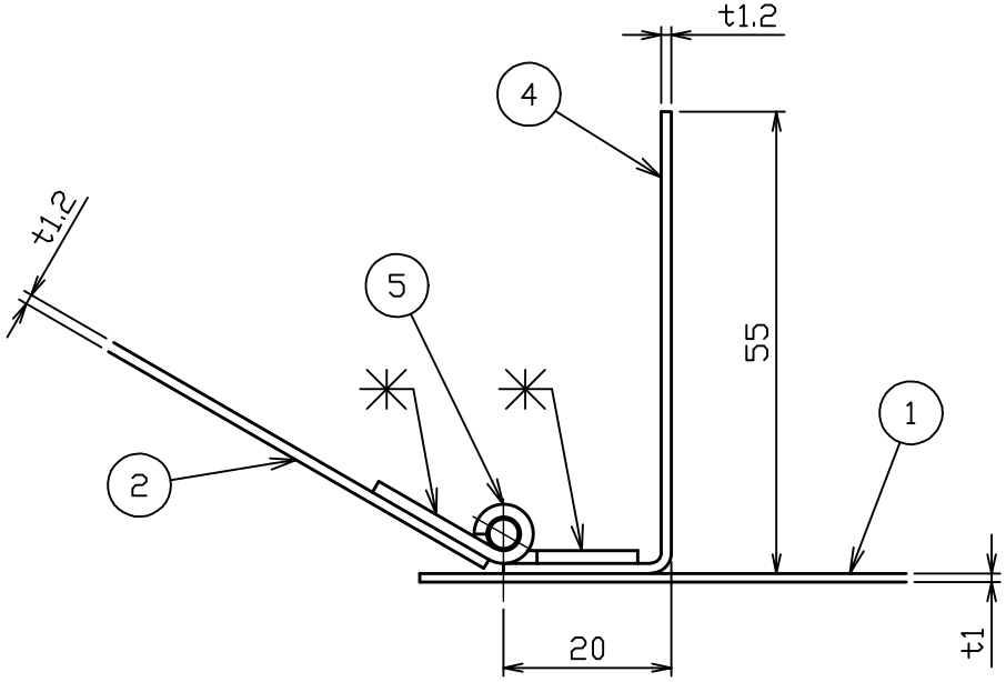
蝶番取付詳細図 S = 1 : 1
