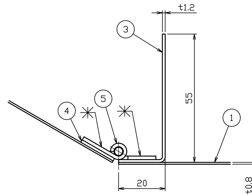
蝶番取付詳細図 S = 1 : 1
