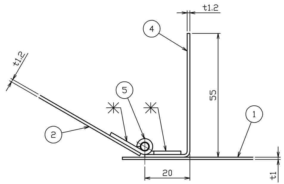
蝶番取付詳細図 S = 1 : 1
