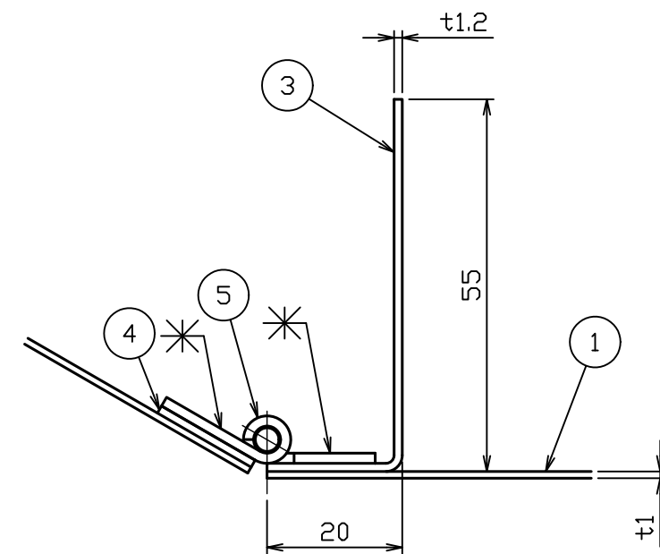
蝶番取付詳細図 S = 1 : 1
