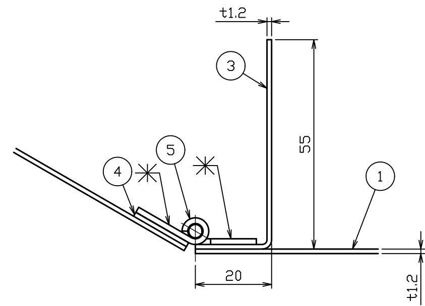
蝶番取付詳細図 S = 1 : 1
